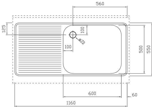
Boven aanzicht
